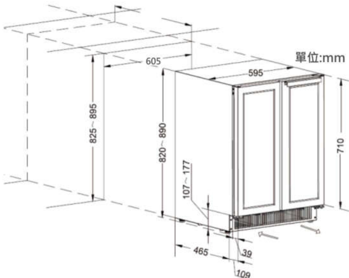
i40DDBE 嵌入式安裝示意圖
